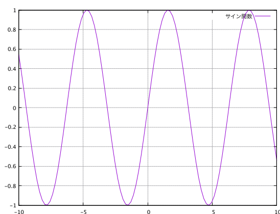
図 2.1 サイン関数のグラフ
